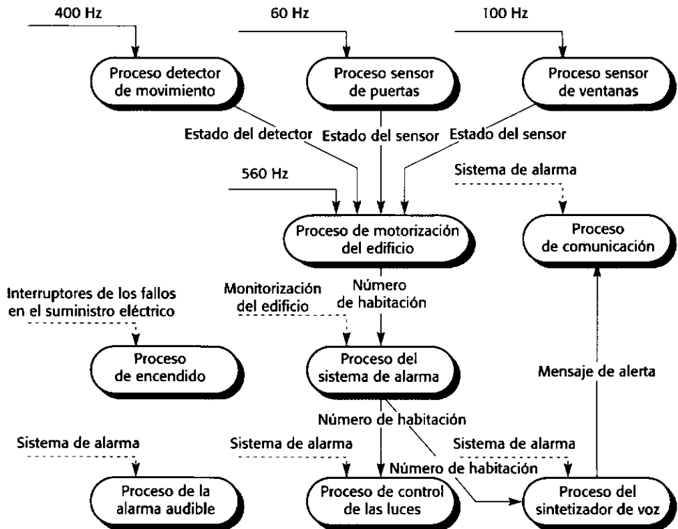
Figura 15.8 Arquitectura de procesos del sistema de alarma antirobo.
