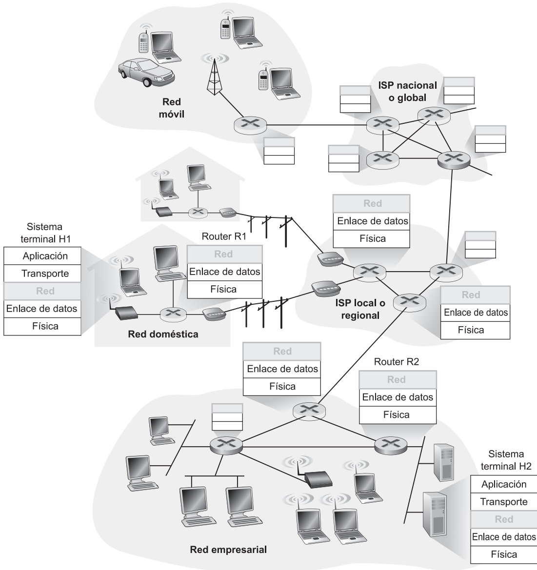
Figura 4.1 • La capa de red.
