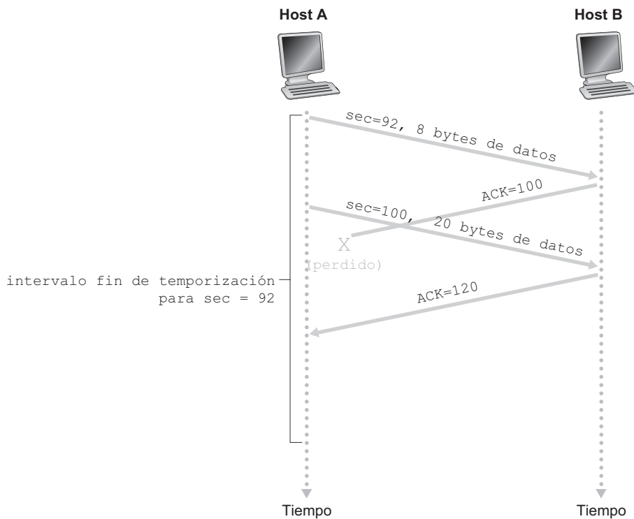
Figura 3.36 • Un reconocimiento acumulado evita la retransmisión del primer segmento.
