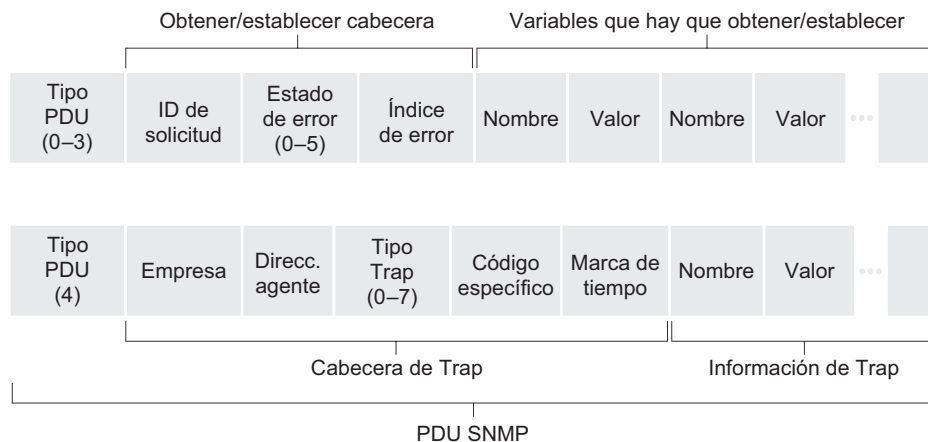
Figura 9.4 • Formato de la PDU de SNMP.
