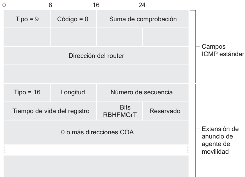
Figura 6.27 • Mensaje de descubrimiento de router ICMP con la extensión de anuncio de agente de movilidad.
