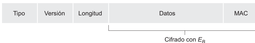
Figura 8.27 • Formato de registro para SSL.
