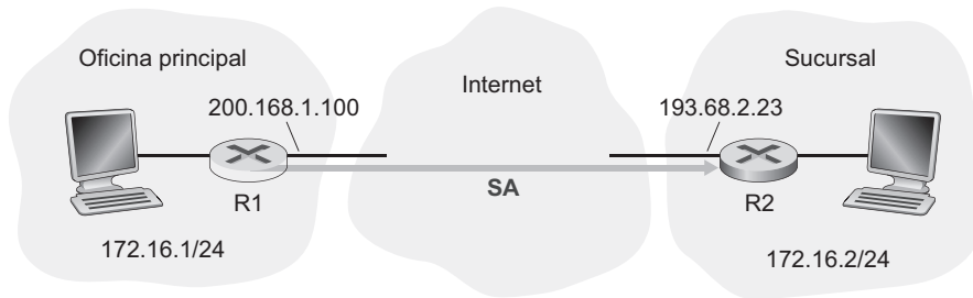
Figura 8.29 • Asociación de seguridad (SA) de R1 a R2.
