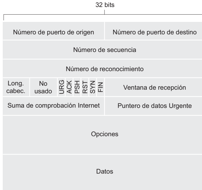
Figura 3.29 • Estructura del segmento TCP.
