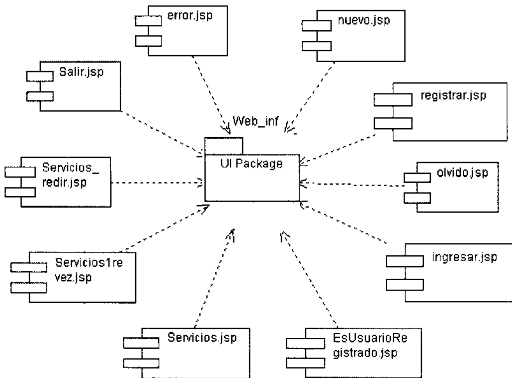
Figura 5. Diagrama de componente.
