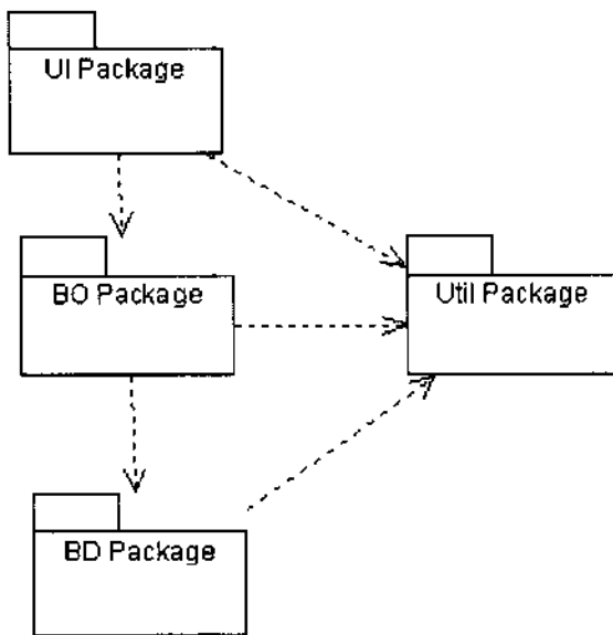
Figura 4. Diagrama de paquetes.
