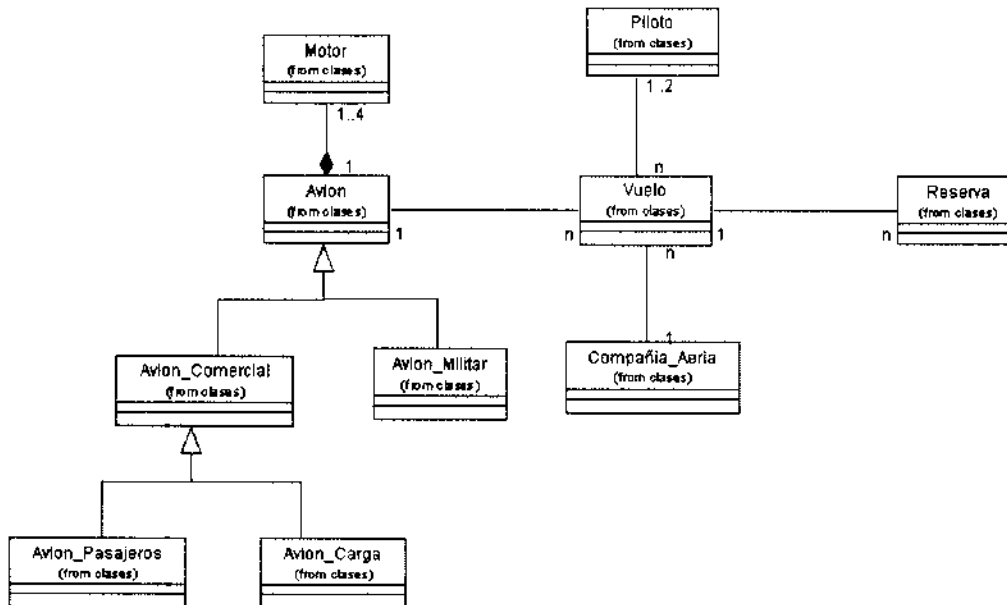
Figura 1. Diagrama de clases.
