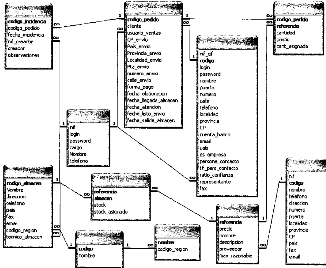
Figura 2. Diseño Lógico de la Base de Datos.
