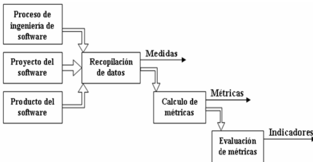
Figura 2. Proceso de recopilación de Métricas del Software
